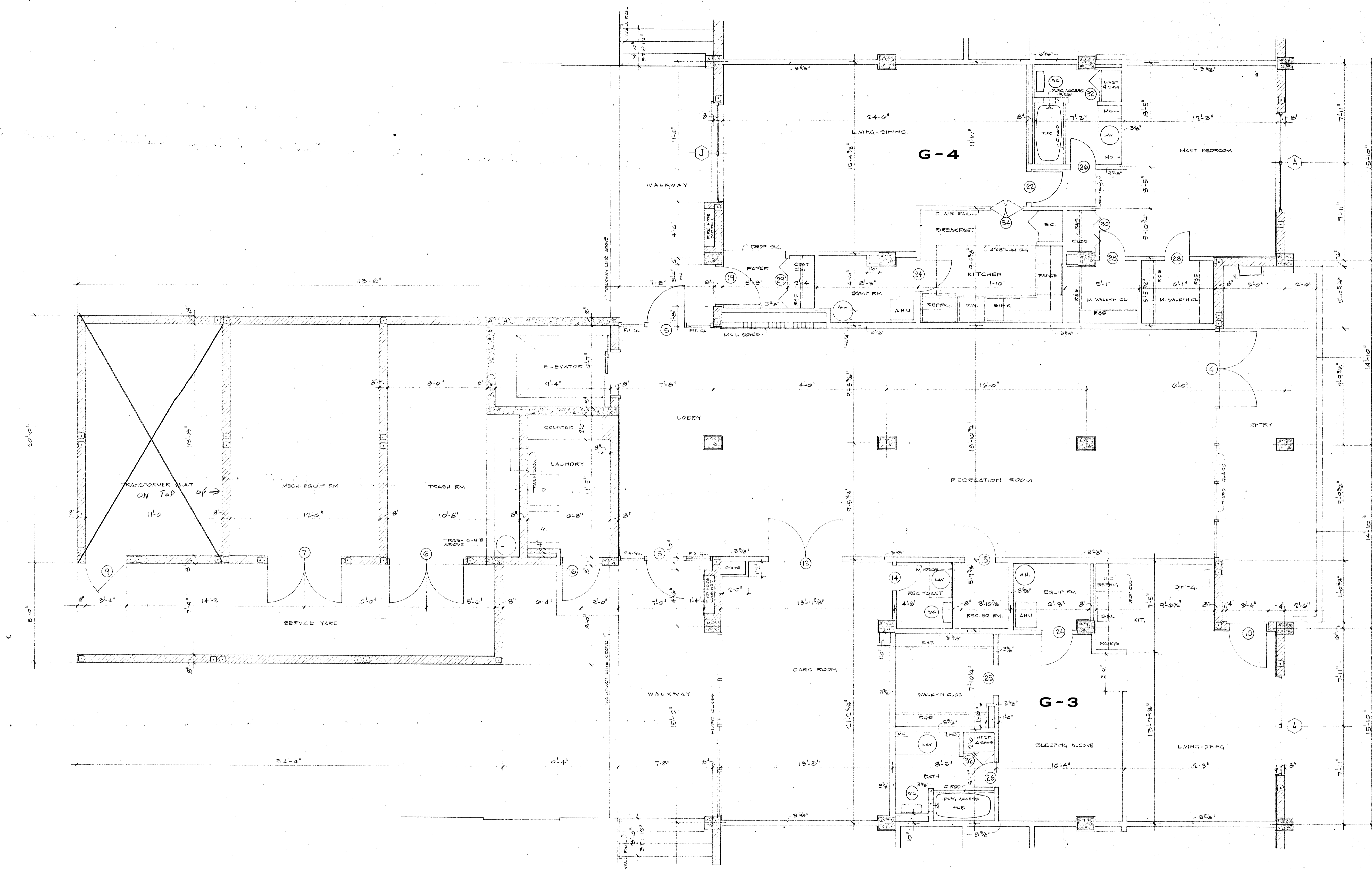
P A R T I A L O R I G I N A L P L A N S C A L E 1/4" = 1'-0"
