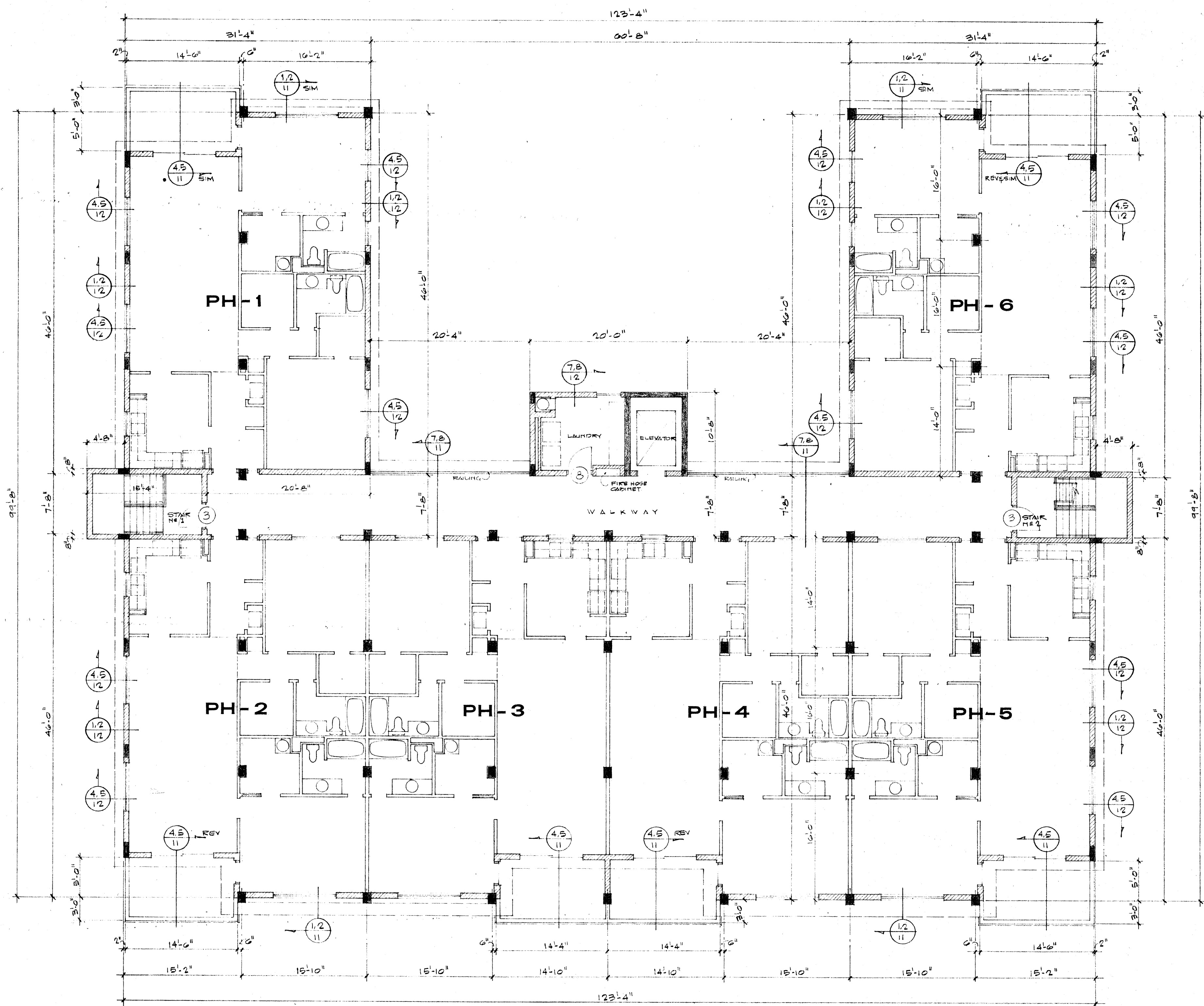
P E N T H O U S E F L O O R P L A N SCALE 1/8" = 1'-0"
