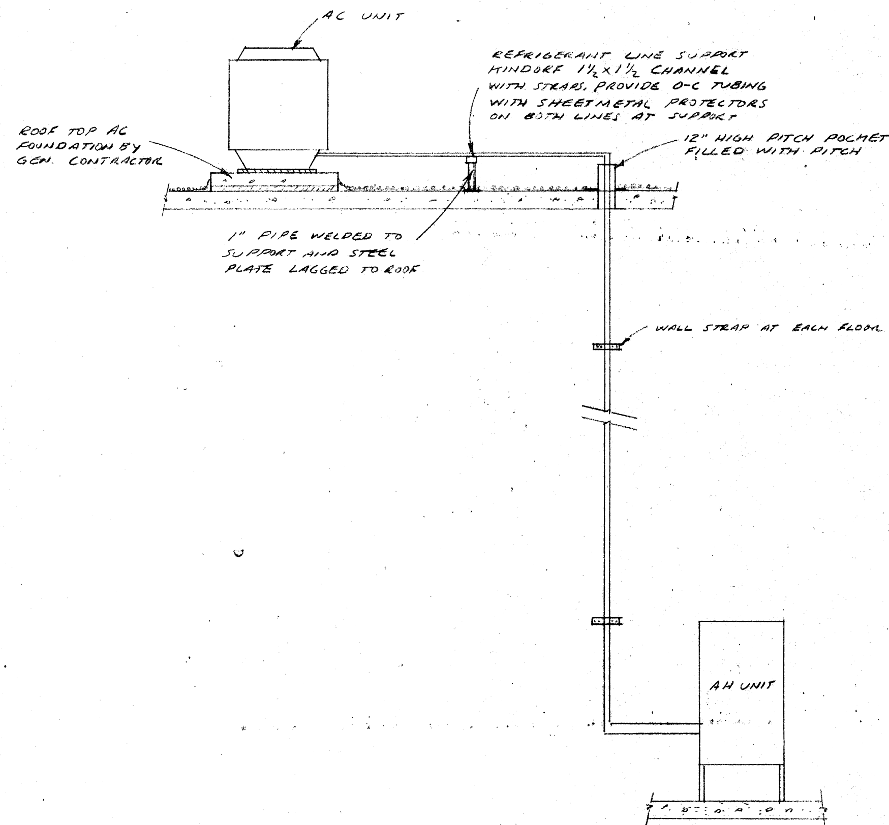
ROOF TOP REFRIGERANT PIPING N.T.S.
